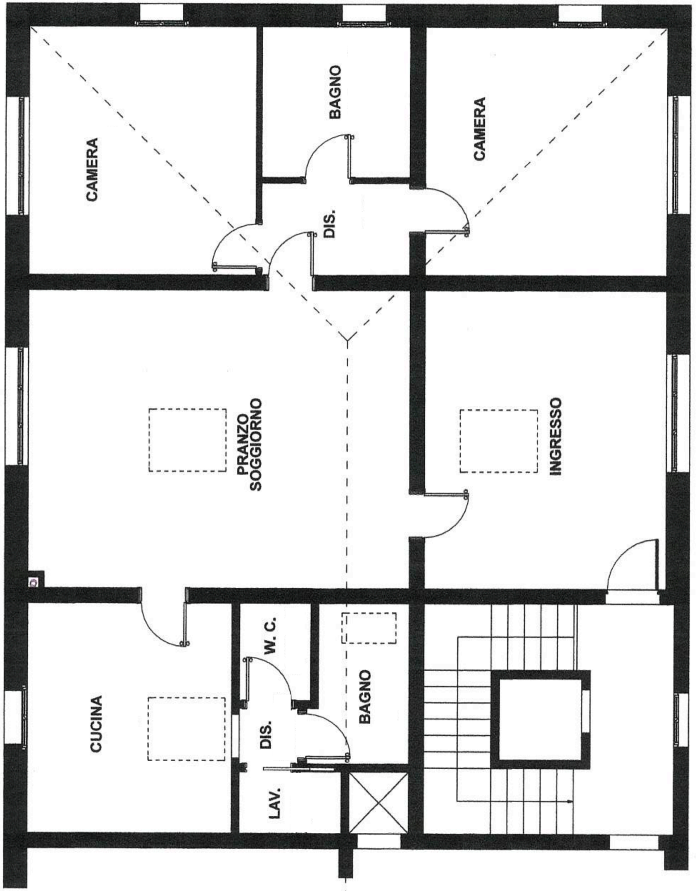
PIANO SECONDO
